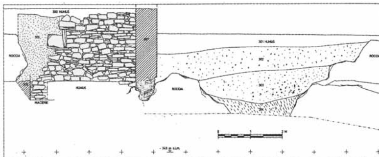
Figura 39- Sezione di rilievo dello scavo archeologico eseguito presso l'abitato di Corvara (da Cagnana A. et Alii, 2008; disegno Landi).
