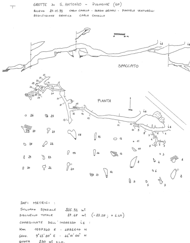
Figura 30 - La Grotta di Sant'Antonio (1065 LI SP) e la Grotta Lunga di Sant'Antonio (1063 LI SP) rilevate nel novembre 1993 da Carlo Cavallo, Sergio Grigoli e Manuela Venturelli (disegno di Carlo Cavallo).
