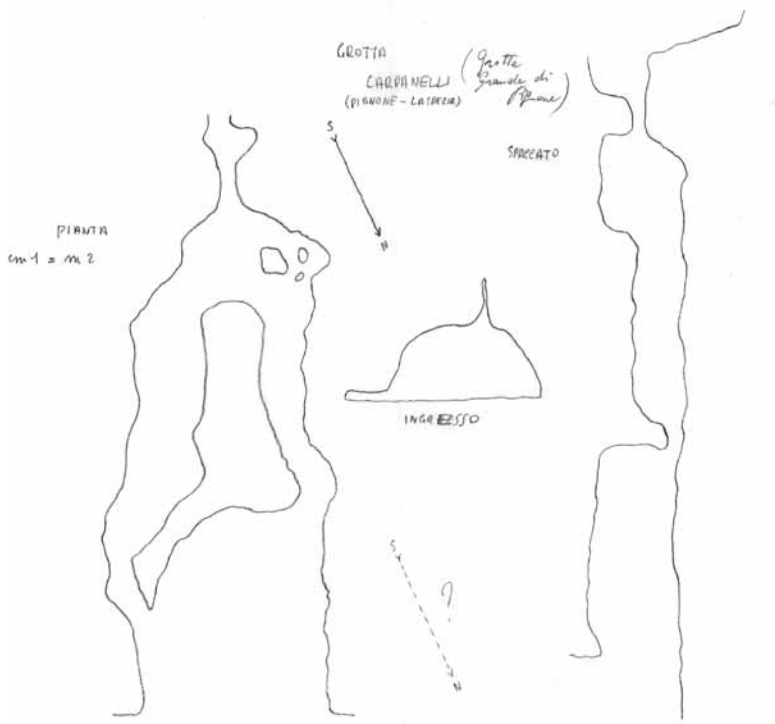
Figura 32 - Schizzo di pianta e sezioni (ingresso e "spaccato") della Grotta Carpanelli, poi Grotta Grande di Pignone (36 LI SP). E' evidente come sia difforme dall'attuale la grande sala di ingresso, evidentemente in un assetto precedente alla coltivazione dell'alabastro che vi è stata praticata.
