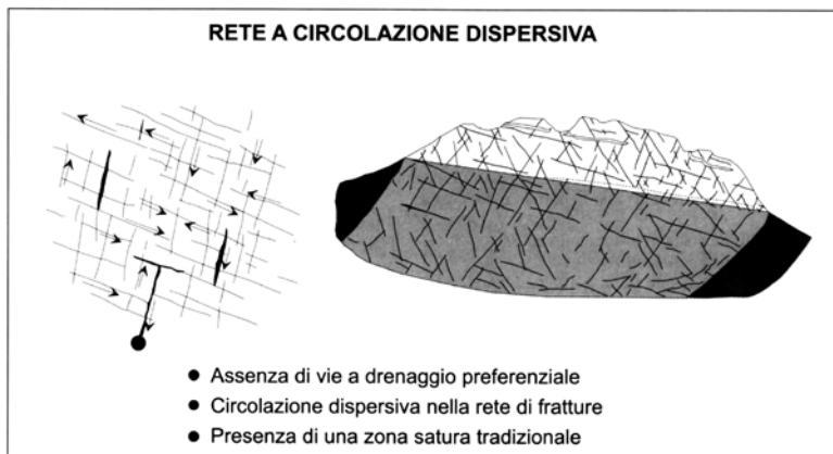
Figura 15 - Rappresentazione schematica di un sistema di drenaggio del tipo “rete a circolazione dispersiva” (da Vigna B. e Calandri G., 2001).
