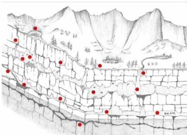
Figura 11 – Spaccato verticale schematico di un sistema carsico. Legenda: 1- rete di fessure, giunti di strato e diaclasi che determina il grado di permeabilità in grande; 2- giunto di strato beante ampliato per corrosione; 3- diaclasi capillare; 4- conca chiusa, dolina; 5- inghiottitoio; 6- pozzo, 7- galleria; 8- grotta; 9- corso d'acqua sotterraneo effimero o stagionale; 10- corso d'acqua sotterraneo perenne; 11- Chirotteri; 12- guano e fauna guanofila; 13- deposito di sabbia e fauna interstiziale; 14- pareti e stalattiti con fauna troglobia; 15- torrente con fauna di acque correnti. Disegno di Patrizia Giannini.
