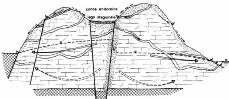
Figura 3.8 – Schema di circolazione idrica sotterranea in acquiferi carbonatici.
