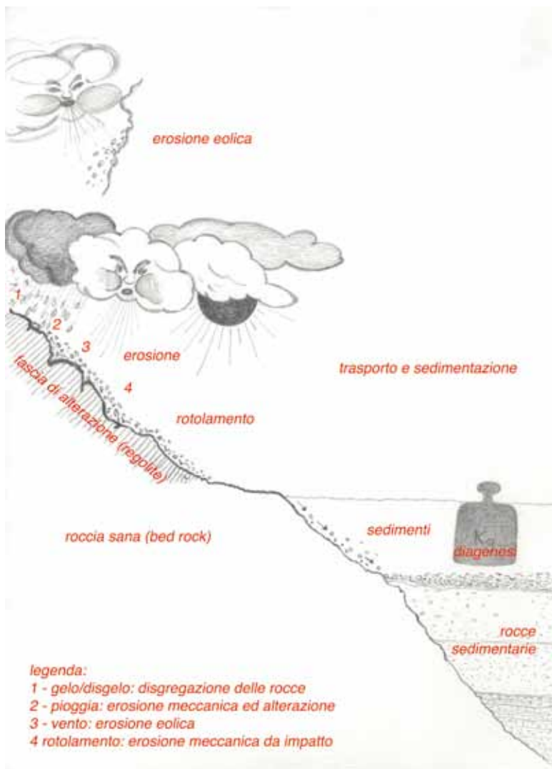
Figura 5 - Rappresentazione schematica dei processi di erosione, trasporto e sedimentazione. Disegno di Patrizia Giannini.
