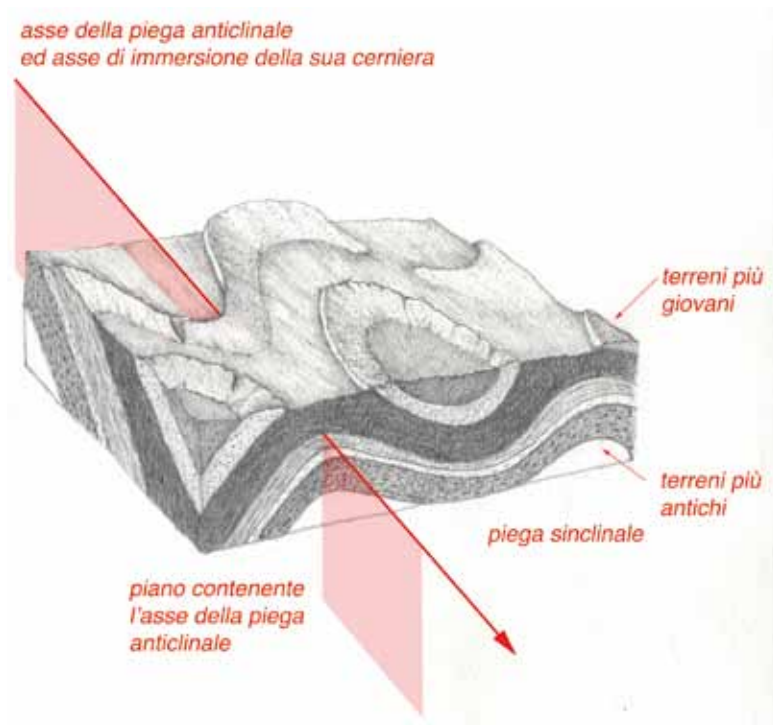
Figura 6 - Schema e nomenclatura di una piega (disegno di Patrizia Gianini).
