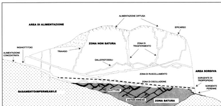
Figura 13 - Rappresentazione schematica e nomenclatura di un acquifero carsico (da Vigna B. e Calandri G., 2001).
