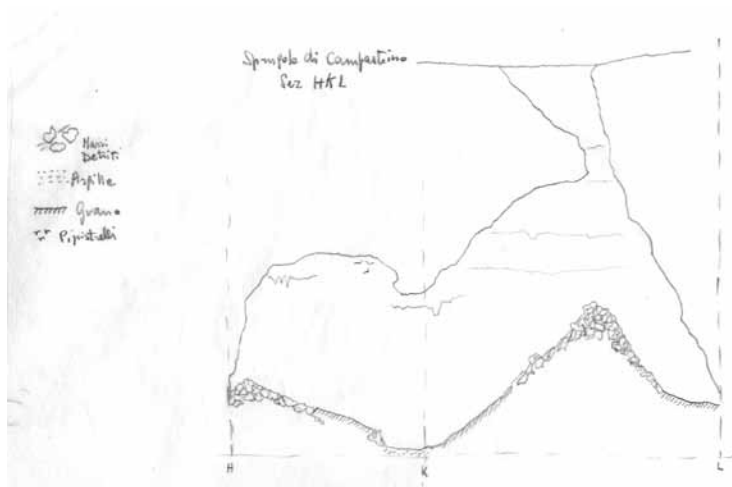
Figura 44 - Sezione principale della Sprugola di Campastrino (192 LI SP) disegnati da Frasca (senza data) alla scala originale di 1:500 (Archivio Gruppo Speleologico Issel, p.g.c.).
