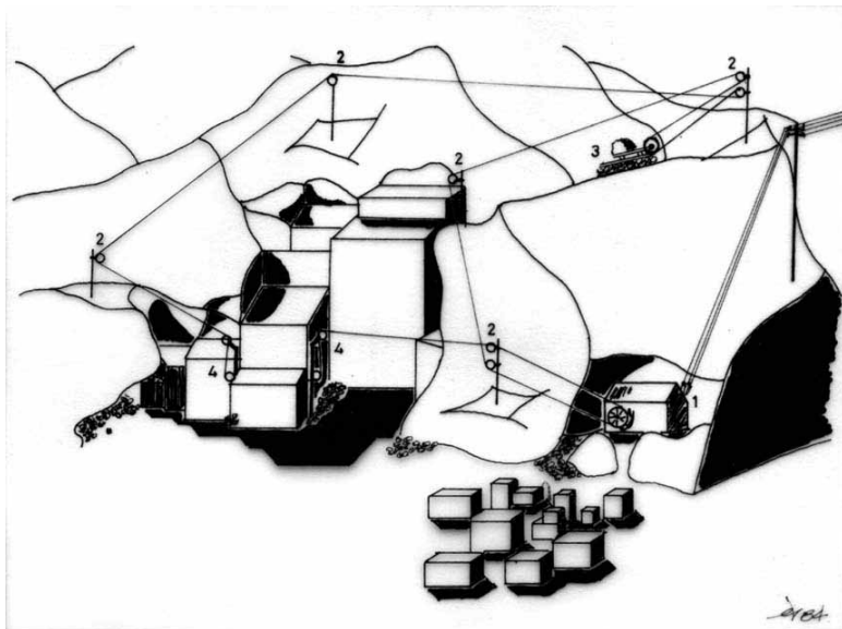
Figura 19 - Il sistema di segazione con filo elicoidale è stato utilizzato nelle cave fino agli anni Ottanta, circa, del secolo scorso. Si trattava di far girare velocemente un cavo di acciaio ritorto a 3 o 5 trefoli, azionato da un motore a scoppio (1), entro alcune pulegge distribuite all'intorno della cava (2). Il cavo era tenuto in tensione da un peso (3) ed in corrispondenza del blocco da tagliare dall'affioramento (4) era utilizzata della sabbia silice ed acqua per velocizzare l'operazione. Disegno di Marco Del Soldato (1984).
