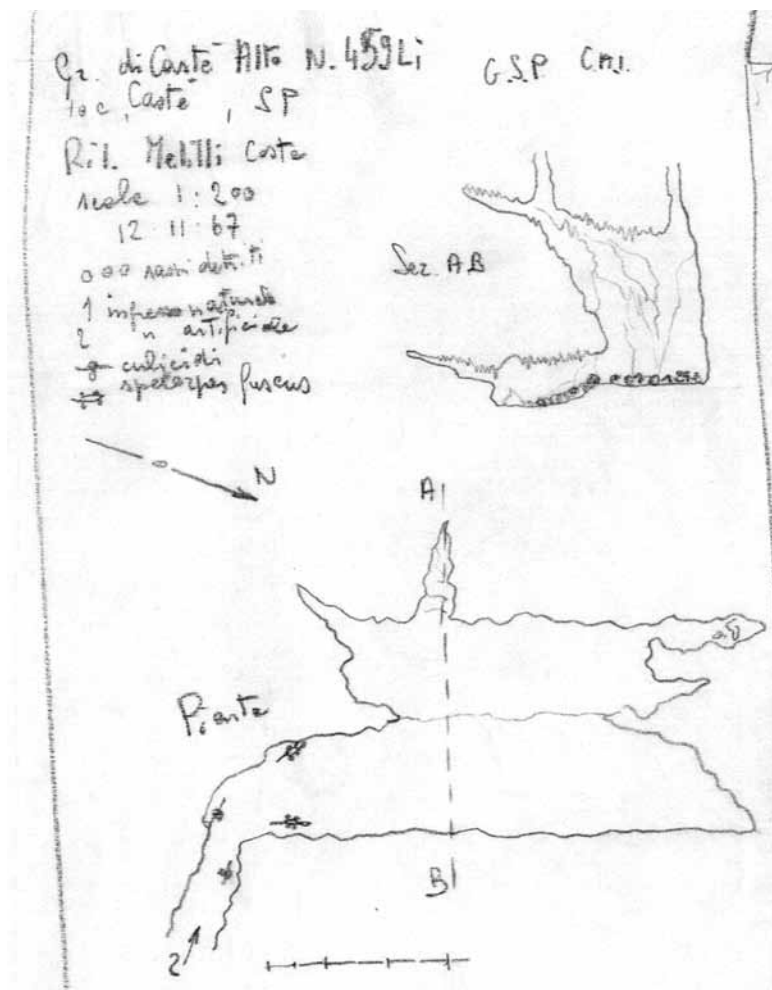
Figura 50 - La Grotta di Castè Alto nella planimetria e sezioni di Melilli e Costa (Archivio del Gruppo Speleologico Issel, p.g.c.).
