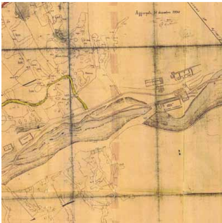
Figura 20 - Particolare del piano interno della miniera manganesifera della Cerchiara, aggiornato al 1930 (archivio privato).
