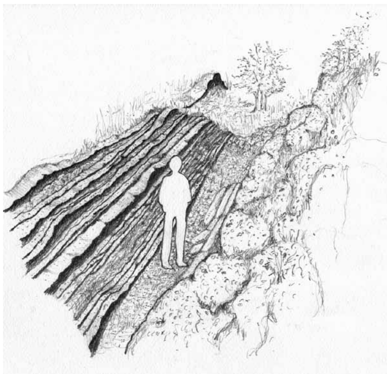
Figura 43 - Il contatto di tipo stratigrafico (cioè che avviene in maniera sfumata) fra i Calcari di Portovenere finemente stratificati ed i Calcari e Marne di Monte Santa Croce , in banchi grossolani e con le superfici fittamente interessate da vaschette di corrosione (tipici Karren semilibri ), nel disegno di Patrizia Giannini.
