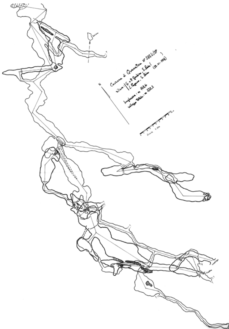
Figura 54 - Rilievo di campagna della Caverna di Quaratica (235 LI SP) eseguito fra l'ottobre ed il novembre 1982 da G. e P. Gerbino, S. Zoia ed L. Pagano (Archivio Gruppo Speleologico Issel, p.g.c.).
