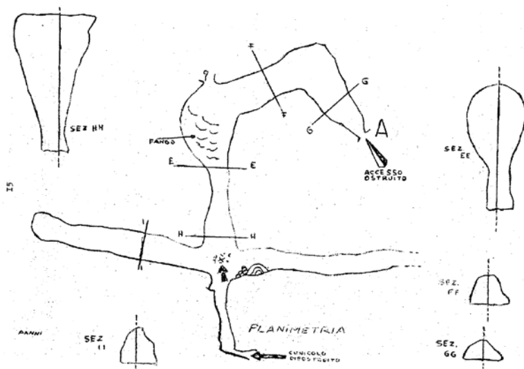
Figura 27 - la Grotta dei Picconi (1611 LI SP) rilevata e disegnata da Andrea Gianni nel 1973-74 (da GIANNI A., 1974).
