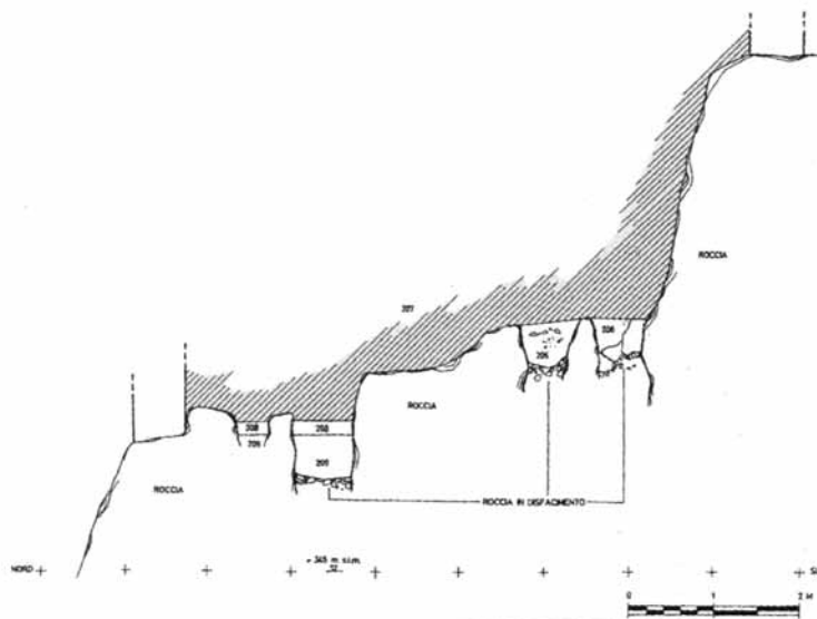
Figura 40 - Sezione di scavo di uno degli edifici medievali di Corvara: 1. roccia carsificata, 2. murature appoggiate o alloggiate nella roccia, che sigillano le fessure riempite di rifiuti (3.) durante la precedente fase di insediamento del sito (da Cagnana A. et Alii, 2008; disegno Landi).
