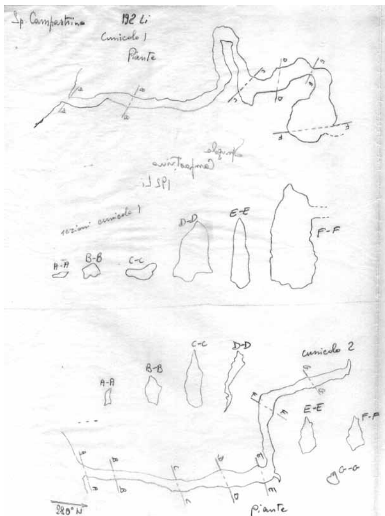
Figura 45 - Cunicoli e relative sezioni della Sprugola di Campastrino (192 LI SP) disegnati da Frasca (senza data) alla scala originale di 1:500 (Archivio Gruppo Speleologico Issel, p.g.c.).
